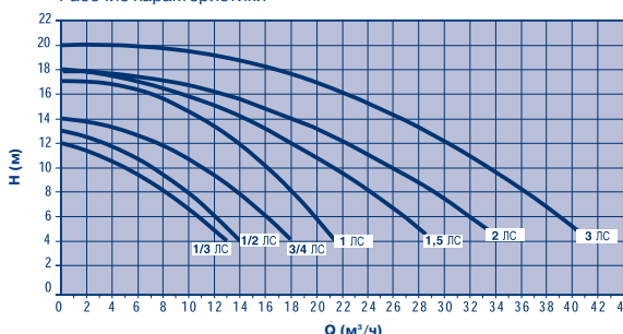
Рабочие характеристики
