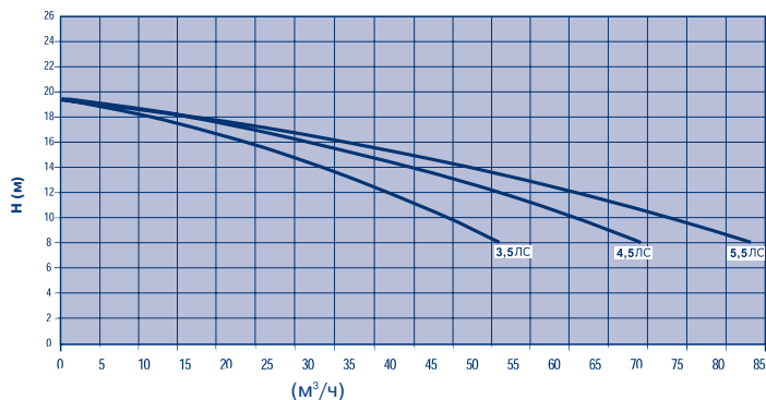
Рабочие характеристики
